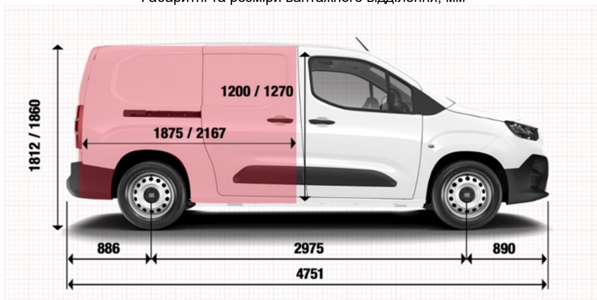
Габаритні та розміри вантажного відділення, мм
